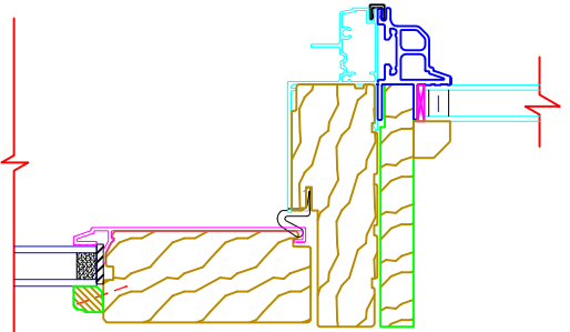
RADIUS / INSWING DOOR 0" Mull Shown W/ OPTIONAL 1", 1 1/4", 2", 3", OR 4"
